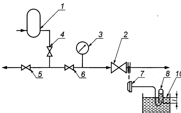
а) схема стэнда для объемного метода контроля герметичности затвора арматуры с проходными корпусами (с патрубками на одной оси и со смещенными осями патрубков)
