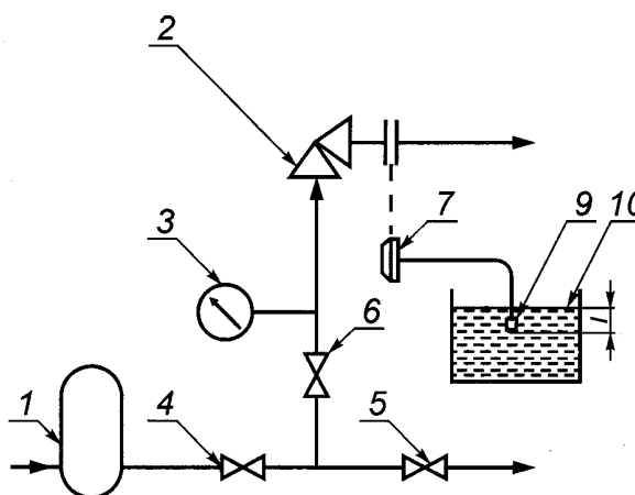
б) схема стэнда для пузырькового метода контроля герметичности затвора арматуры с угловыми корпусами
