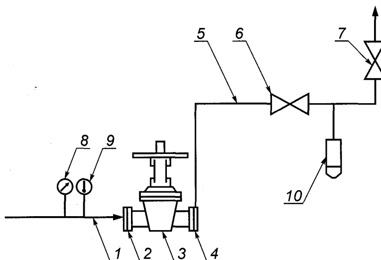
Рисунок Б.1 - Рекомендуемая схема стенда для испытаний арматуры в сборе на прочность и плотность материала корпусных деталей и сварных швов и герметичность относительно внешней среды по подвижным и неподвижным соединениям
