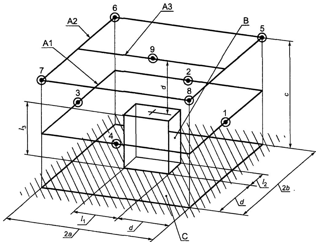
Рисунок С.1 — Точки измерений (согласно рисунку В.2 ГОСТ 31275)
