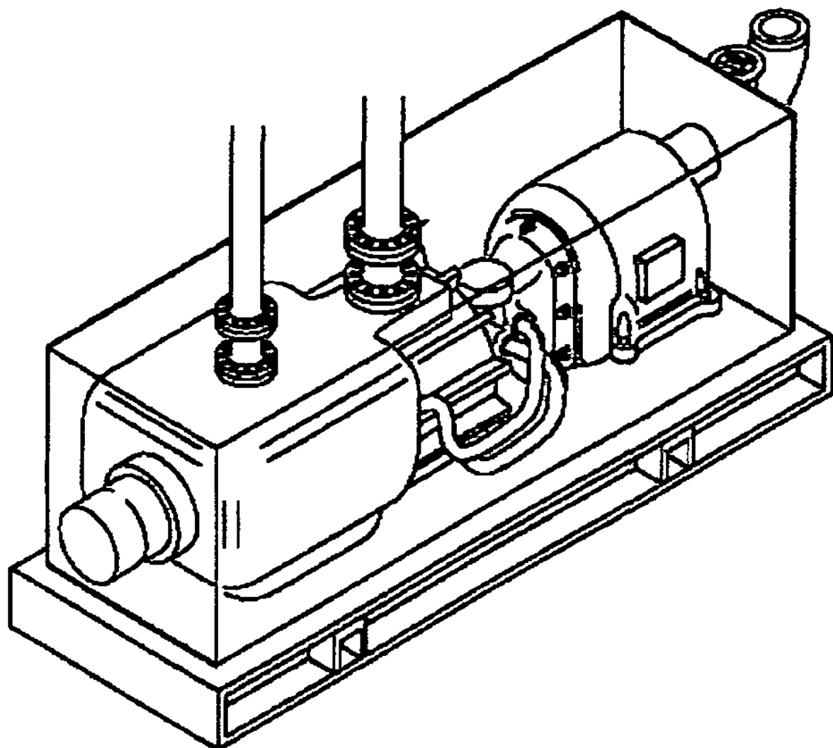
Рисунок Е.3 — Ротационный компрессор
