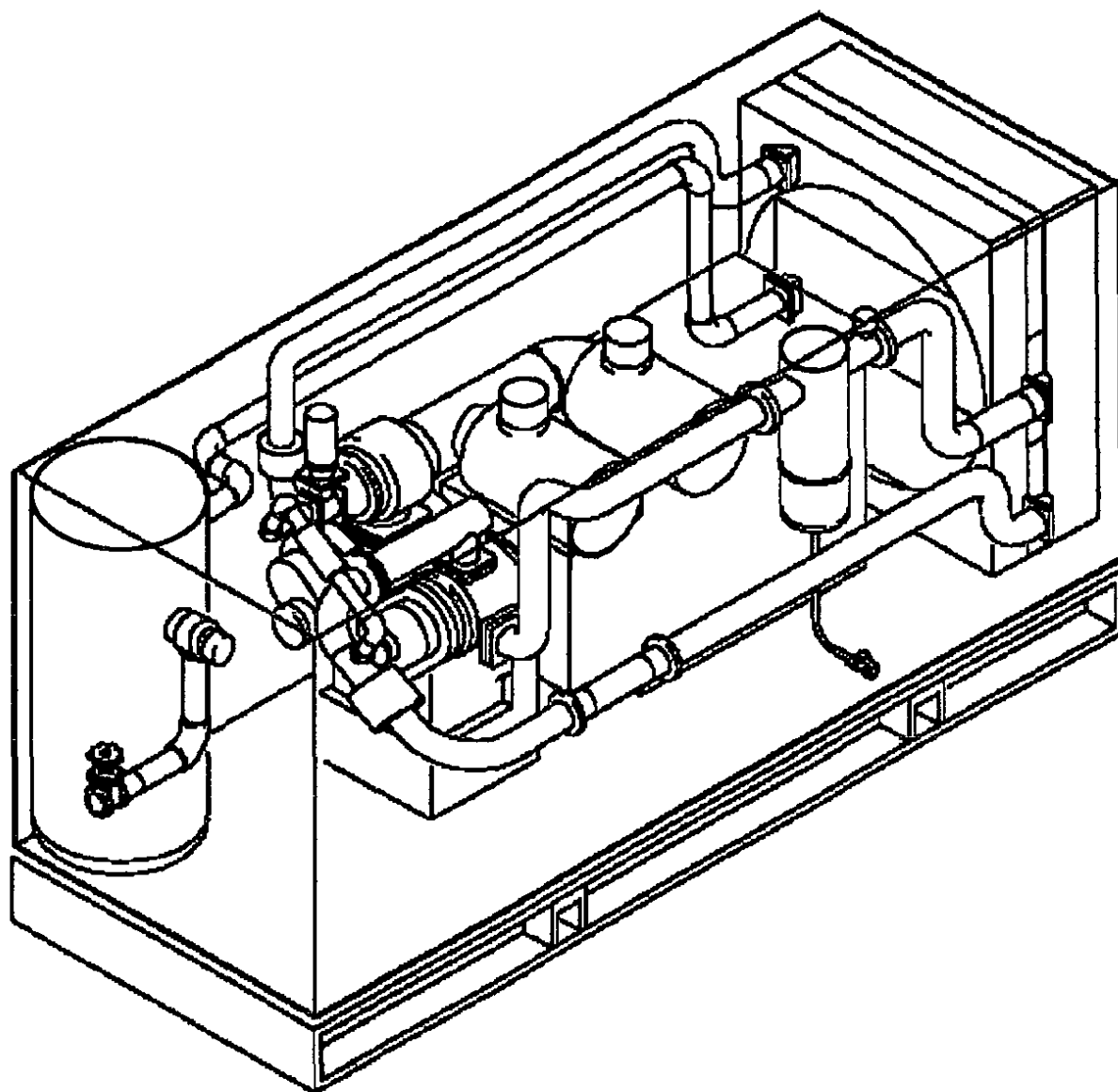
Рисунок Е.1 — Обычный компрессор
